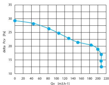
Fan efficiency characteristic Rohrlüfterleistungskennlinie
