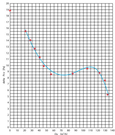
Fan efficiency characteristic Rohrlüfterleistungskennlinie
