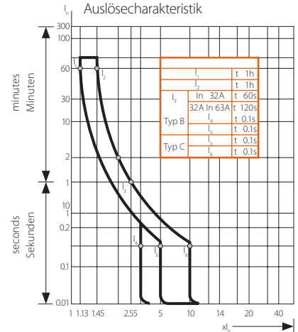
Release characteristic Auslösecharakteristik
